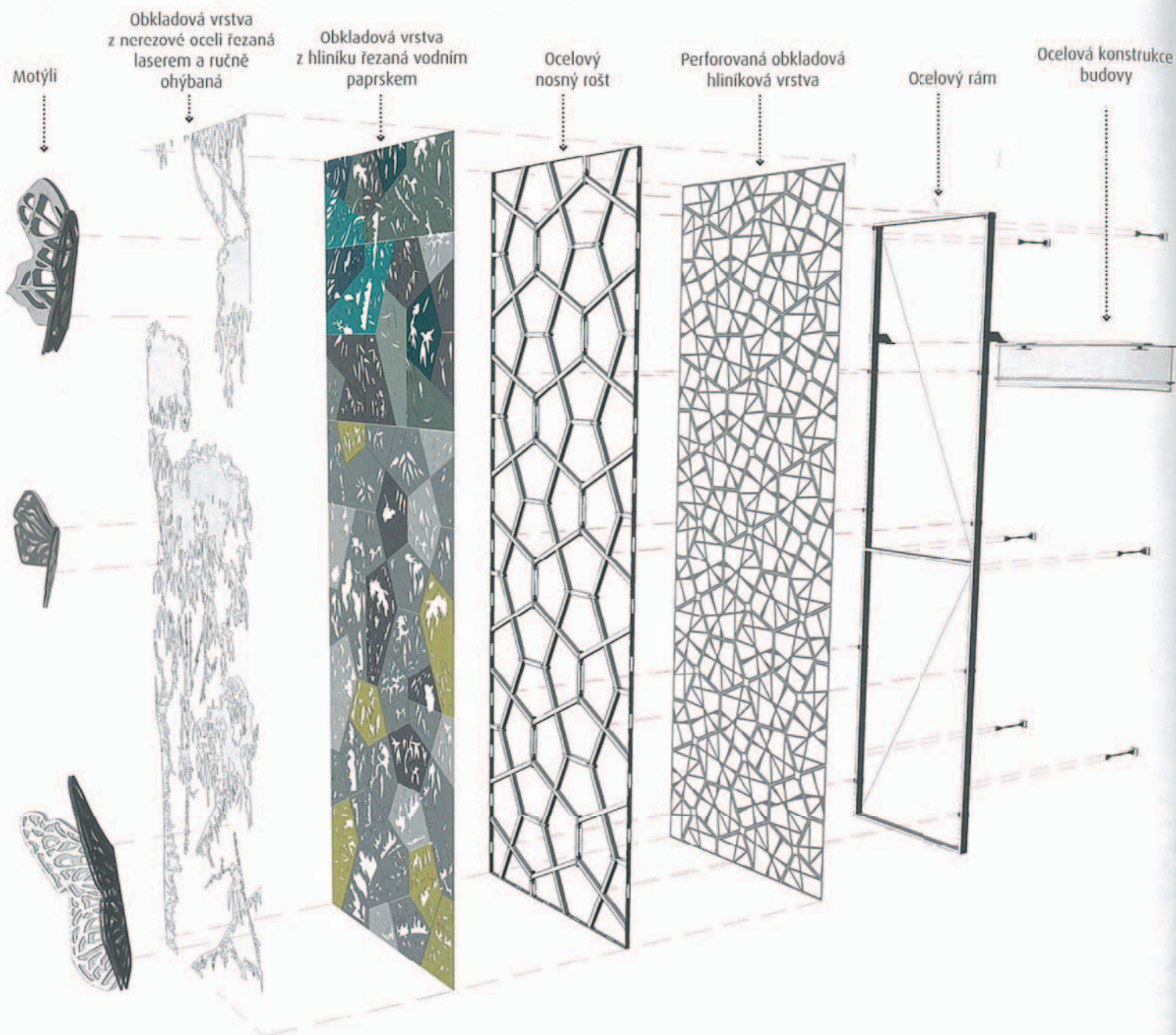
Schéma skladby fasády
